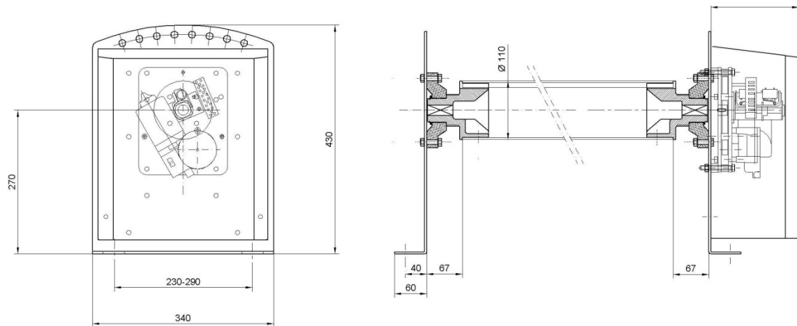
Abbildung 4-1: Ausführung ACOE 45
