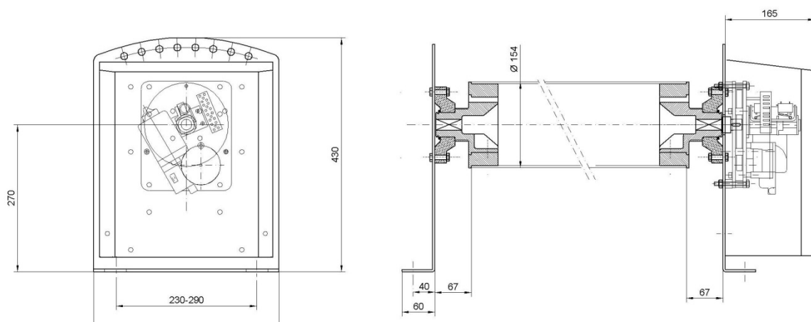
Abbildung 4-2: Ausführung ACOE 50
