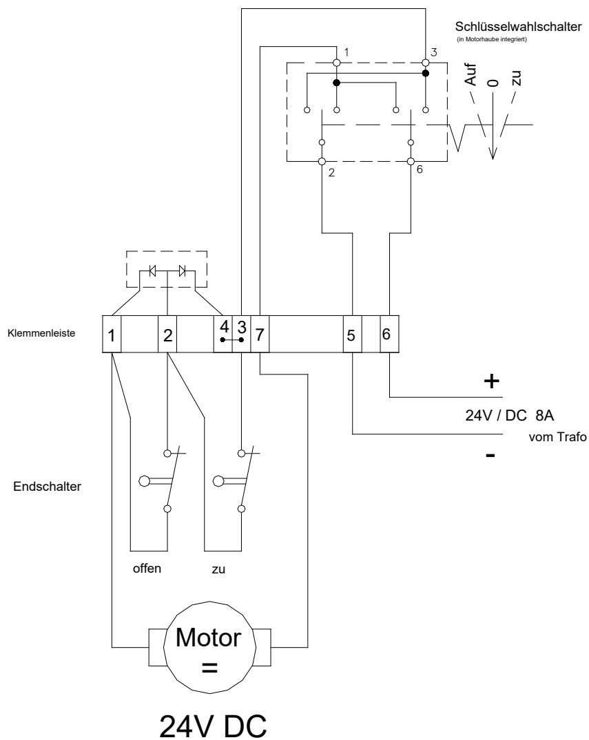
Abbildung 3-2: Anschluß des Schlüsselwählschalters
