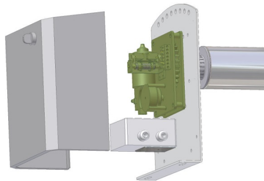
Abbildung 3-6: Ansicht Motor mit Steuerung
